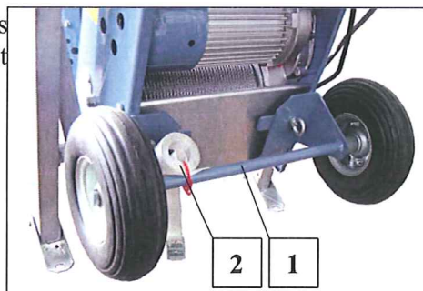
Fig. 13 montera chassi
