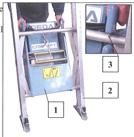
Fig. 31 montera stegvinsch
