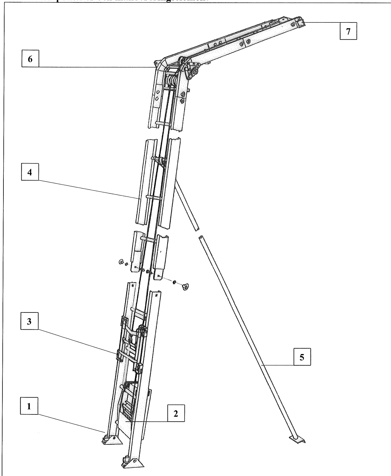
Fig. 4 GEDA-LIFT
