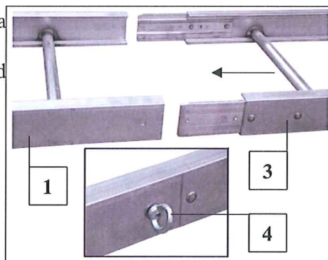
Fig. 19 montera ihop stegdelar
