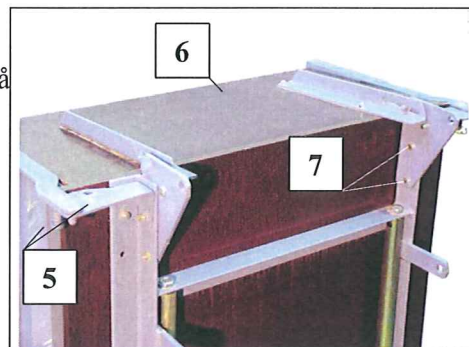
Fig. 45 montera läm varioplattform
