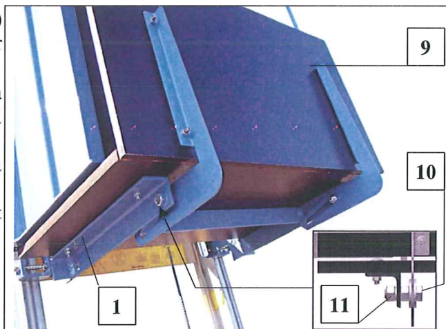
Fig. 41 frontskydd för universalflak
