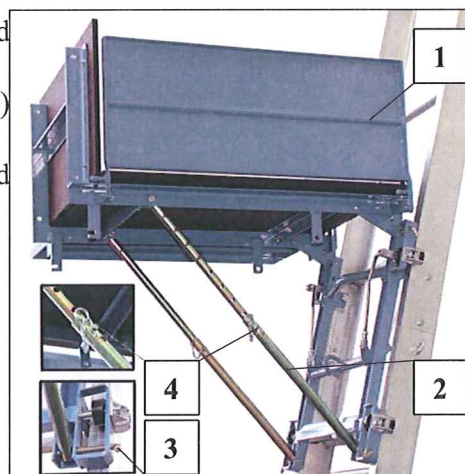
Fig. 47 Vario- Bühne
