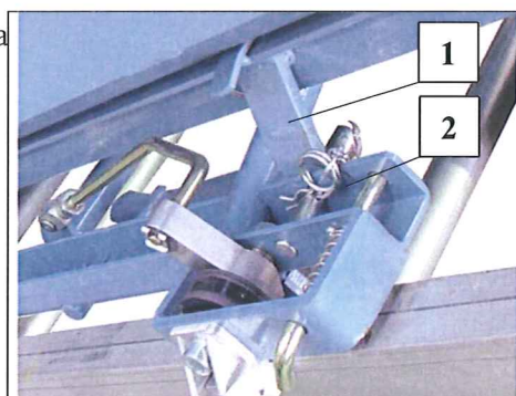
Fig. 59 montera tippskopa
