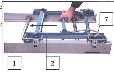
Fig. 18 för in sliden i fotdelen
