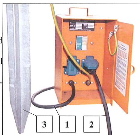
Fig. 17 Liten byggströmsfördelare
