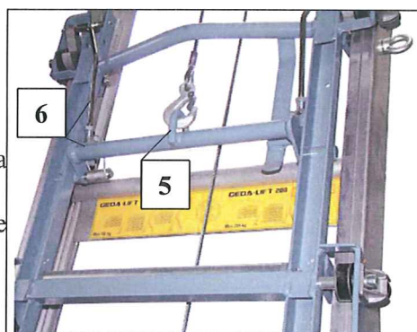
Fig. 38 haka i kabeln på sliden
