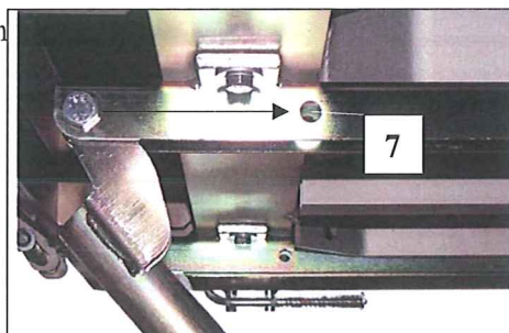
Fig. 52 koppla teleskopstöd
