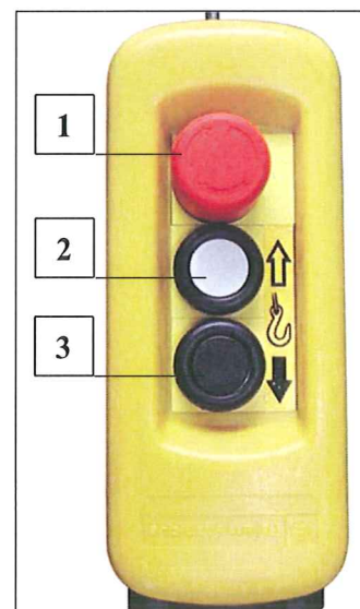
Fig. 71 hankontroll enstegad
