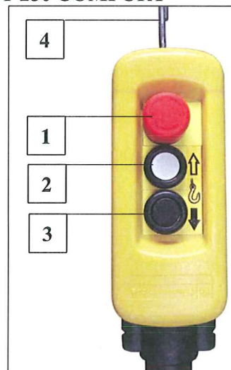
Fig. 8 handkontroll (1-stegad)
