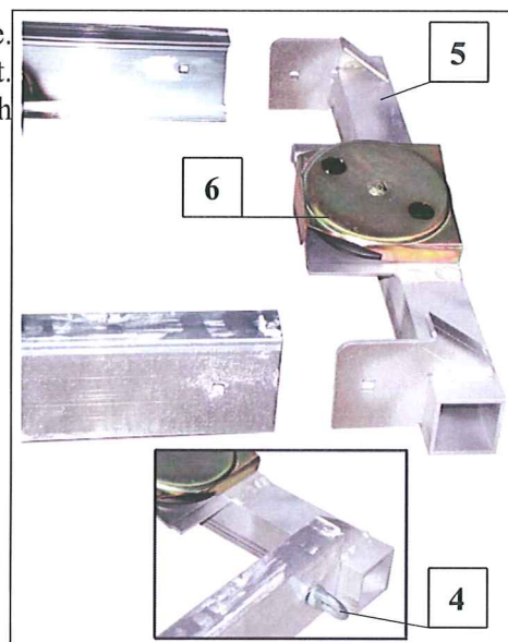
Fig. 20 montera huvudstycke
