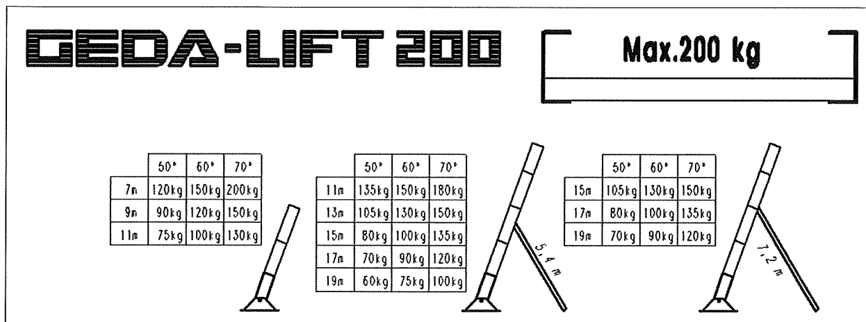
Fig. 24 belastningstabell för stegdelar 150/200 kg
