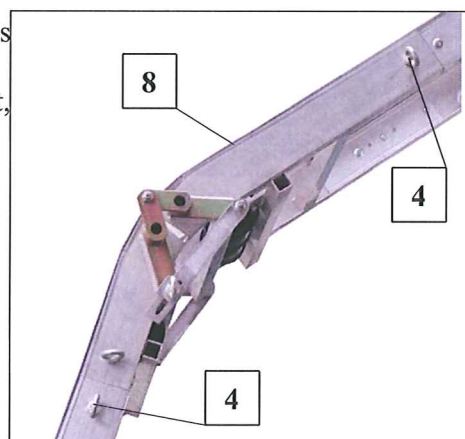
Fig. 21 montera krökstycke
