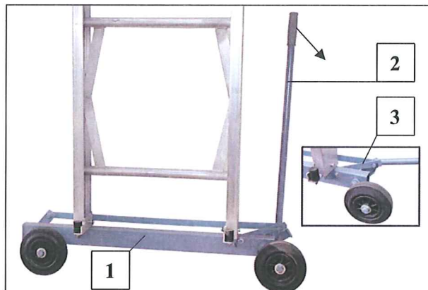
Fig. 14 chassi
