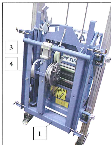
Fig. 63 tippslid
