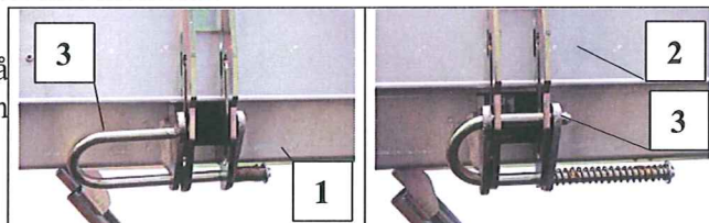
Fig. 49 montera transportplattformens lämmar
