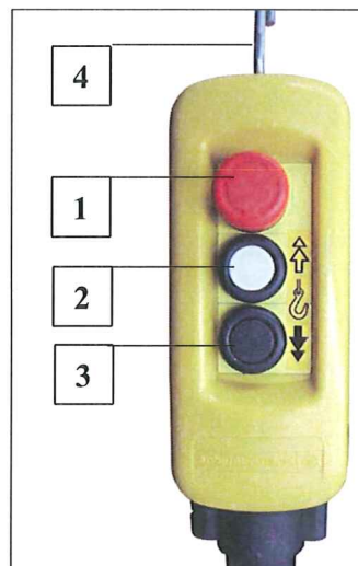
Fig. 9 handkontroll (2-stegad)
