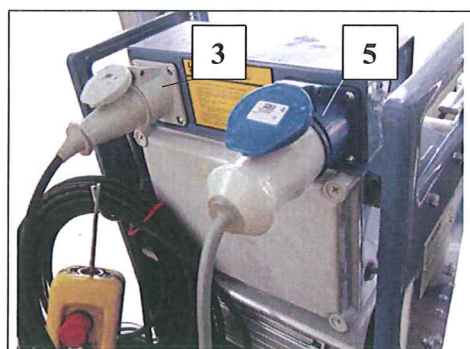
Fig. 7 vinsch FIXLIFT 250
