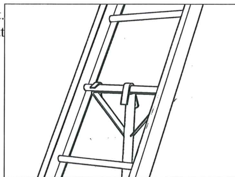
Fig. 28 haka i aluminium-stegstöd
