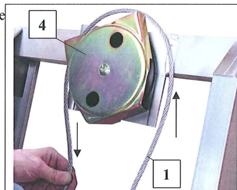
Fig. 35 dra kabeln över huvuddelen
