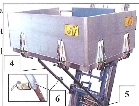
Fig. 51 transportplattform
