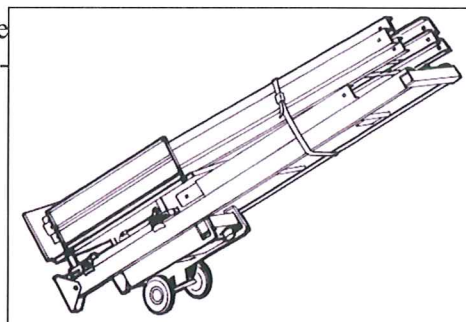
Fig. 12 chassi
