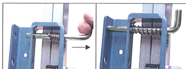
Fig. 39 fjäderregel på slid
