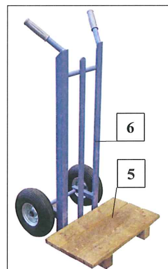
Fig. 57 kärra för taktegelflak
