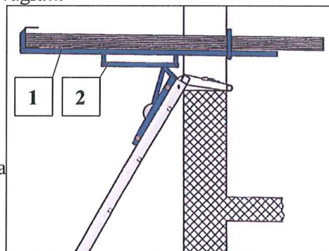
Fig. 68 skivflak med tippslid
