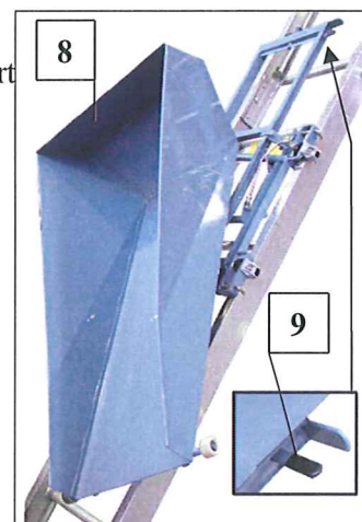
Fig. 62 tömma tippskopan
