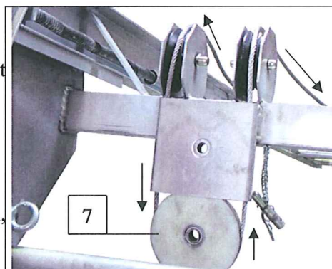
Fig. 61 montera kabeln vid tippanordning
