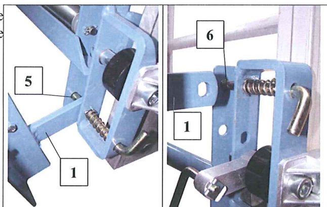
Fig. 42 montera universalflak
