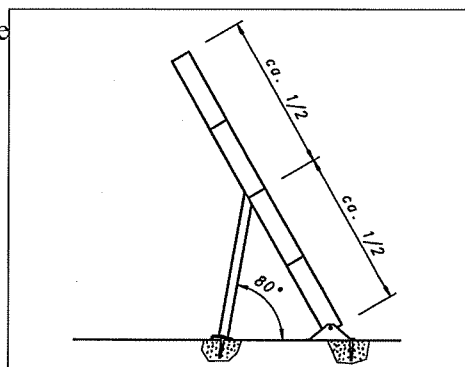
Fig. 30 Stegstödens justeringsvinklar
