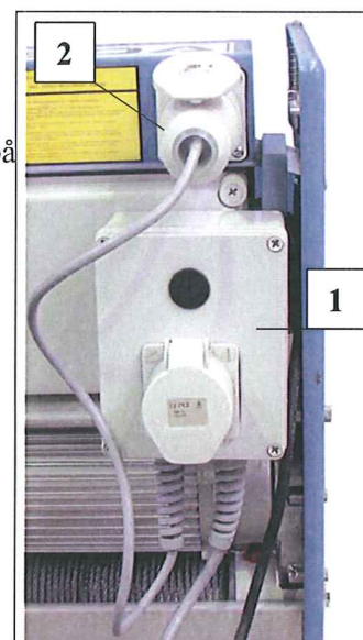
Fig. 69 övergångsstyrning
