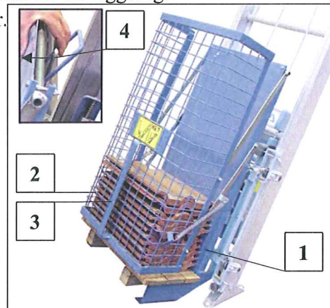
Fig. 56 Taktegelflak
