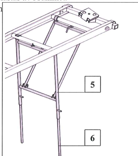
Fig. 55 Stöd för stegbana
