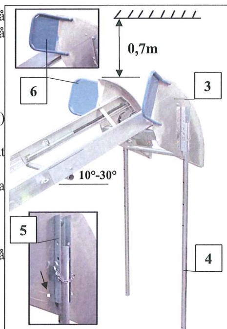
Fig. 60 tippanordning
