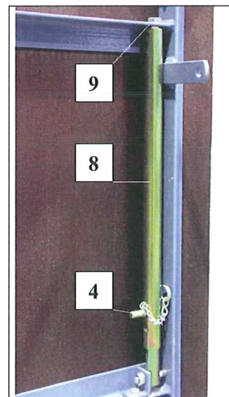
Fig. 46 teleskopstöd vario-plattform
