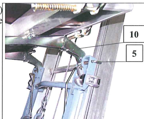
Fig. 50 montera stor transportplattform
