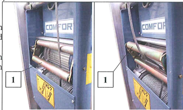
Fig. 11 gränsbrytare nedan
