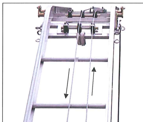
Fig. 37 kabelföring på krökstäck
