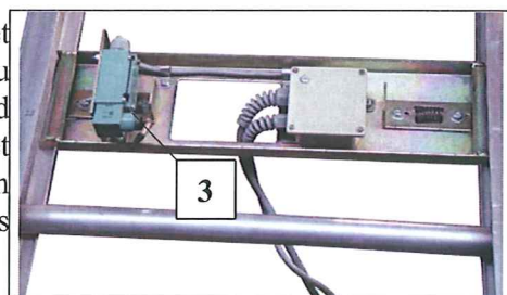
Fig. 70 övergångsbrytare
