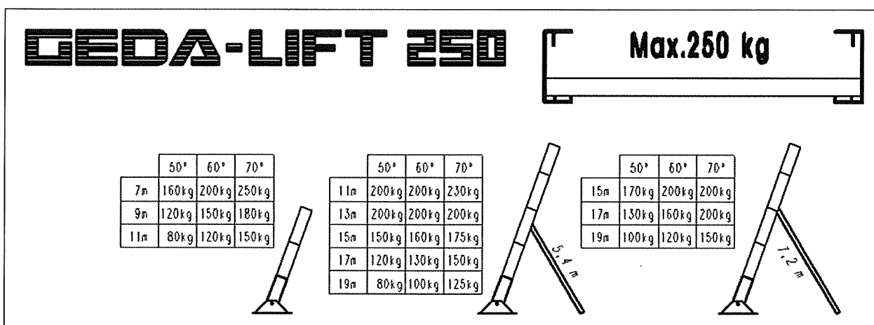
Fig. 25 belastningstabell för stegdelar 200/250 kg
