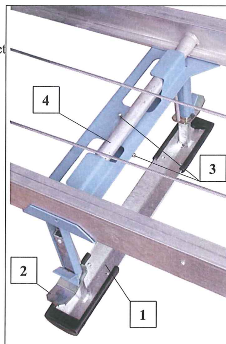
Fig. 15 takstödbock
