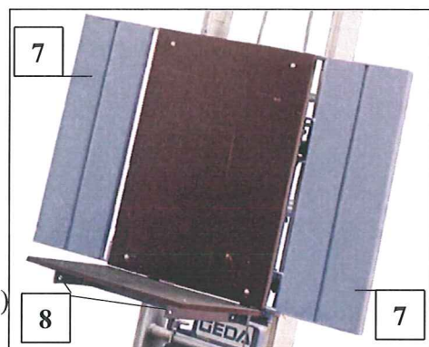
Fig. 43 universalflak
