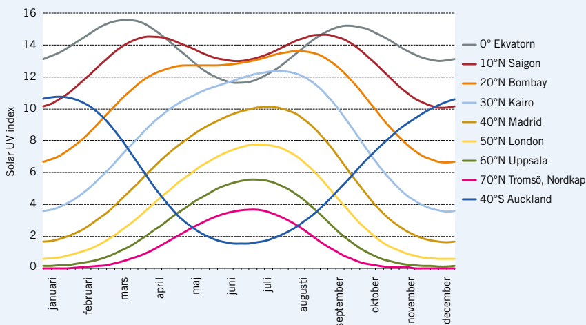
FIGUR 3. Typiska UV-index (ett mått på strålningens styrka) för molnfria dagar och genomsnittlig tjocklek på ozonskiktet skiljer sig kraftigt mellan olika breddgrader på jorden och varierar även under året. På alla platser, även nära ekvatorn, varierar givetvis UV-index under dagen bland annat beroende av solens höjd över marken och molnighet.
