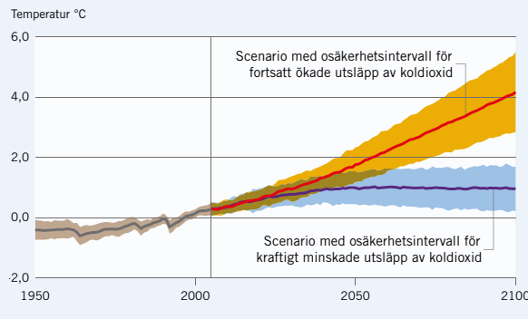
FIGUR 1 Scenarier för global medeltemperatur (jämfört med referensperioden 1986–2005)
