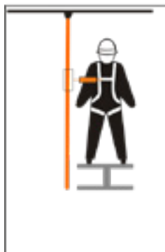
Absorbedor de impacto deslizando con guía móvil
