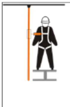
Mitlaufendes Auffanggerät mit beweglicher Führung
