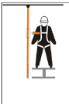
Système d'arrêt de chute de type guidé
